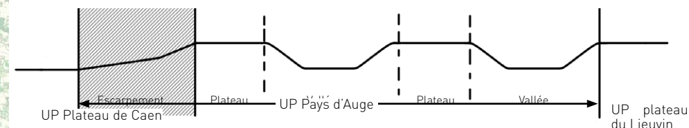
Coupe transversale de principe des structures paysagères des Plateaux et vallées encaissées du Pays d'Auge.
