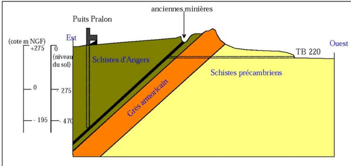
Figure 9 : Coupe géologique schématisée de la formation ferrifère à La Ferrière-aux-Étangs (d'après panneau d'exposition – commune de La Ferrière-aux-Étangs).
