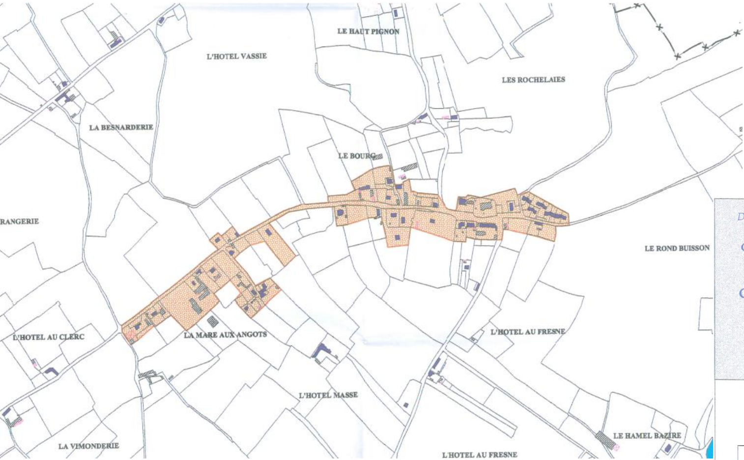
Figure n°1 : Zonage d'assainissement de Cavigny approuvé en 2006
