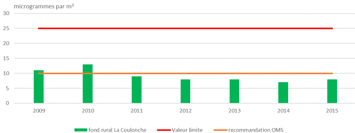
Evolution des moyennes annuelles en PM2.5 dans le département de l'Orne
