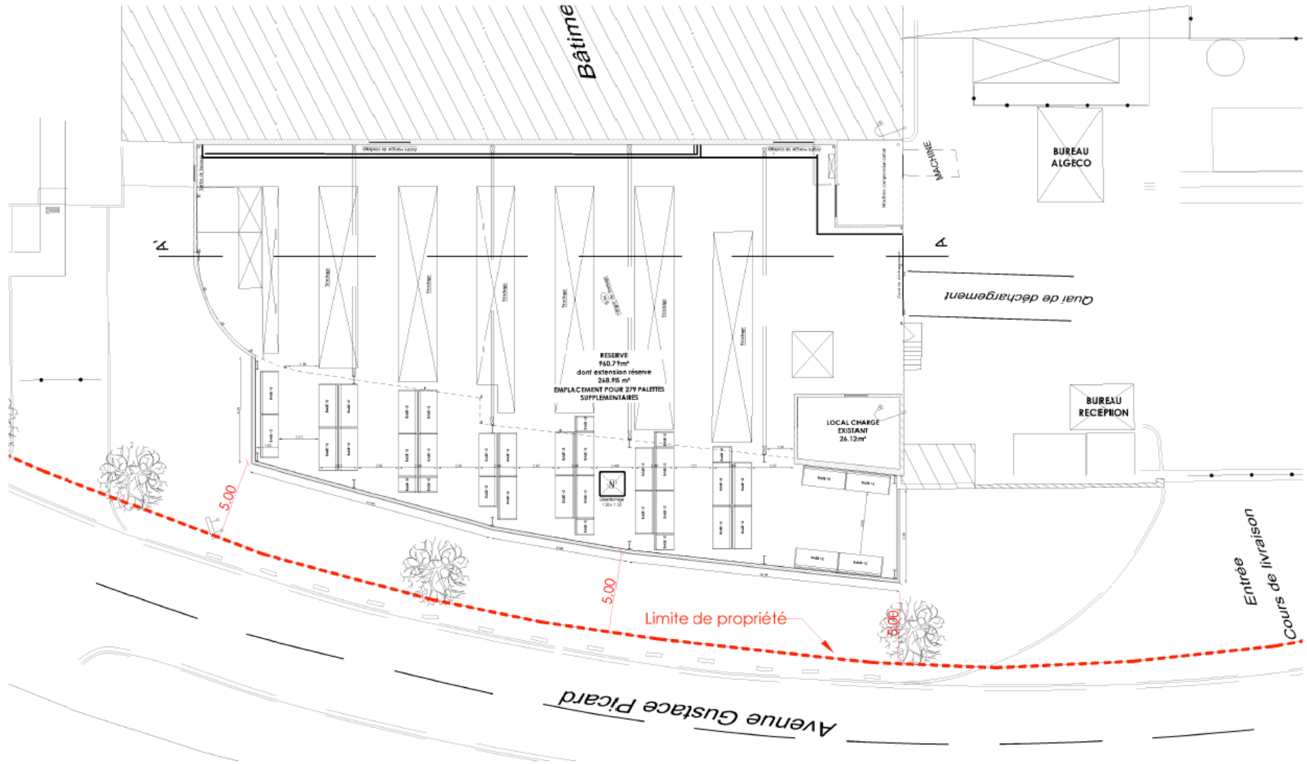
Plan masse projet 2/2 (source : Marraud Ingénierie)
