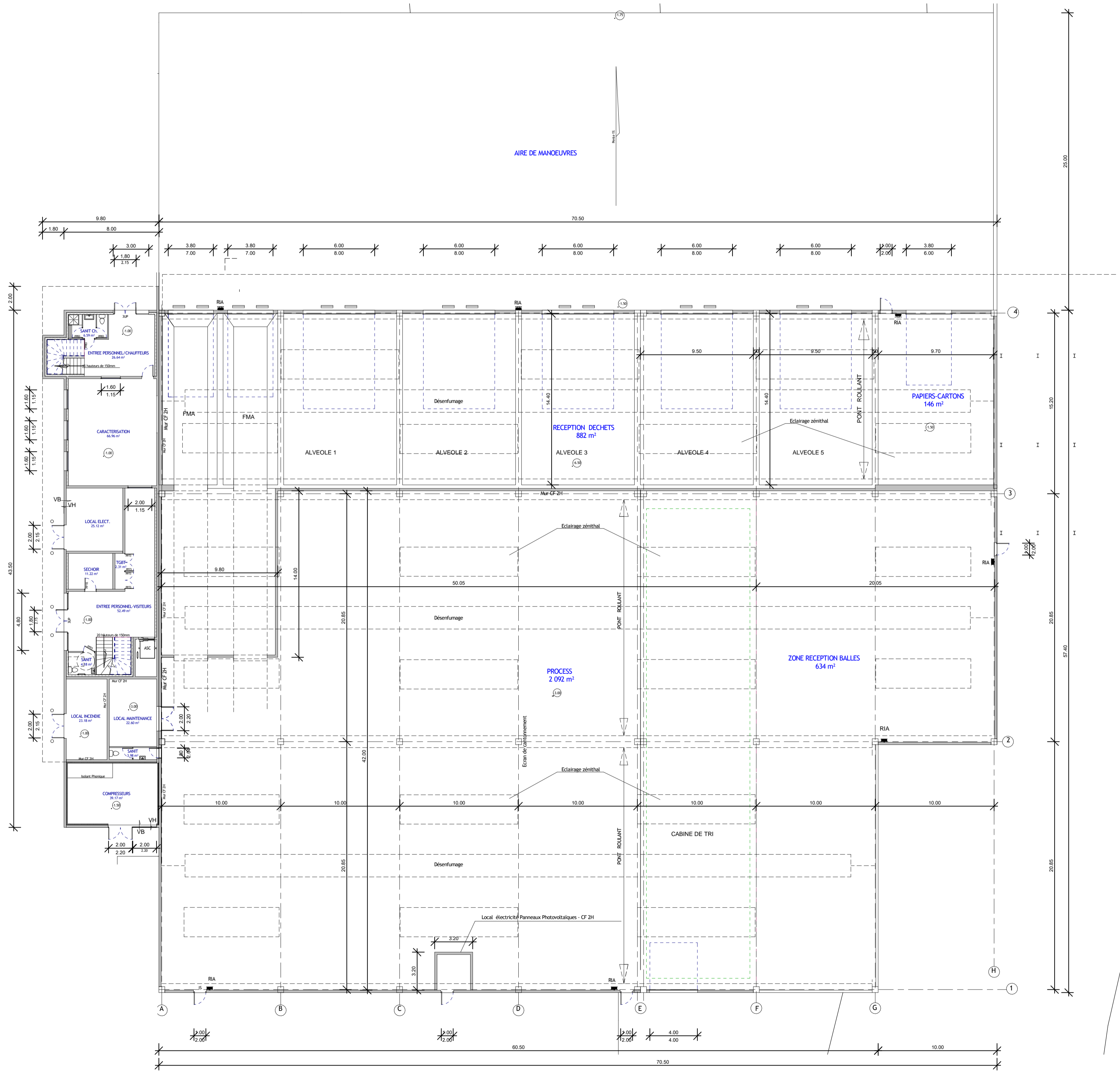
R 0 - LOCAUX TECHNIQUES SURFACE DE PLANCHER : 4 070 m 2 SURFACE UTILE : 4 037 m 2
