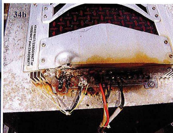
Figure 34 : Balise sonore testée à Chausey par le groupe de travail en 2007 (34a), peu résistante dans ce type de milieu (34b).
