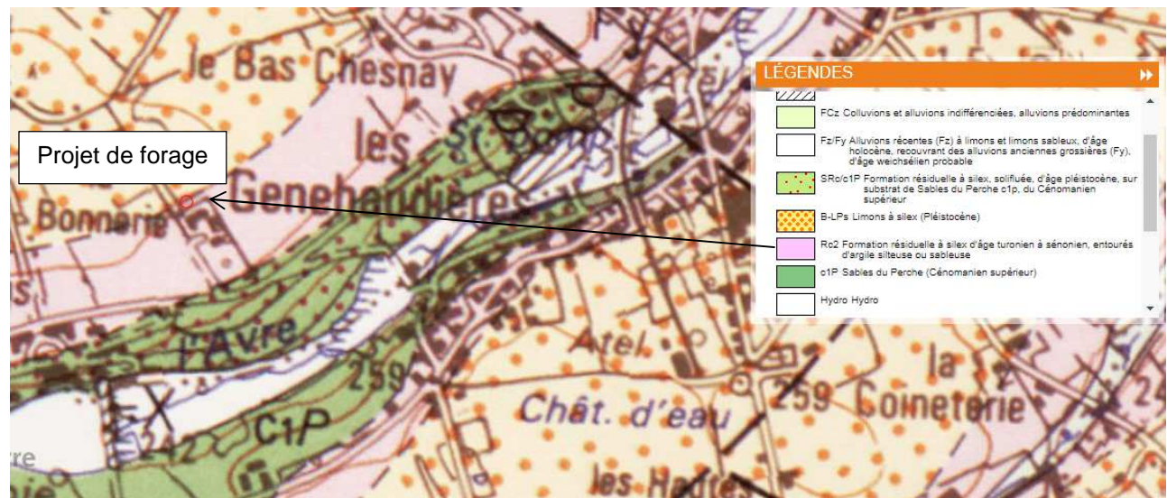
Carte géologique (Source : Infoterre.brgm.fr, 2020)
