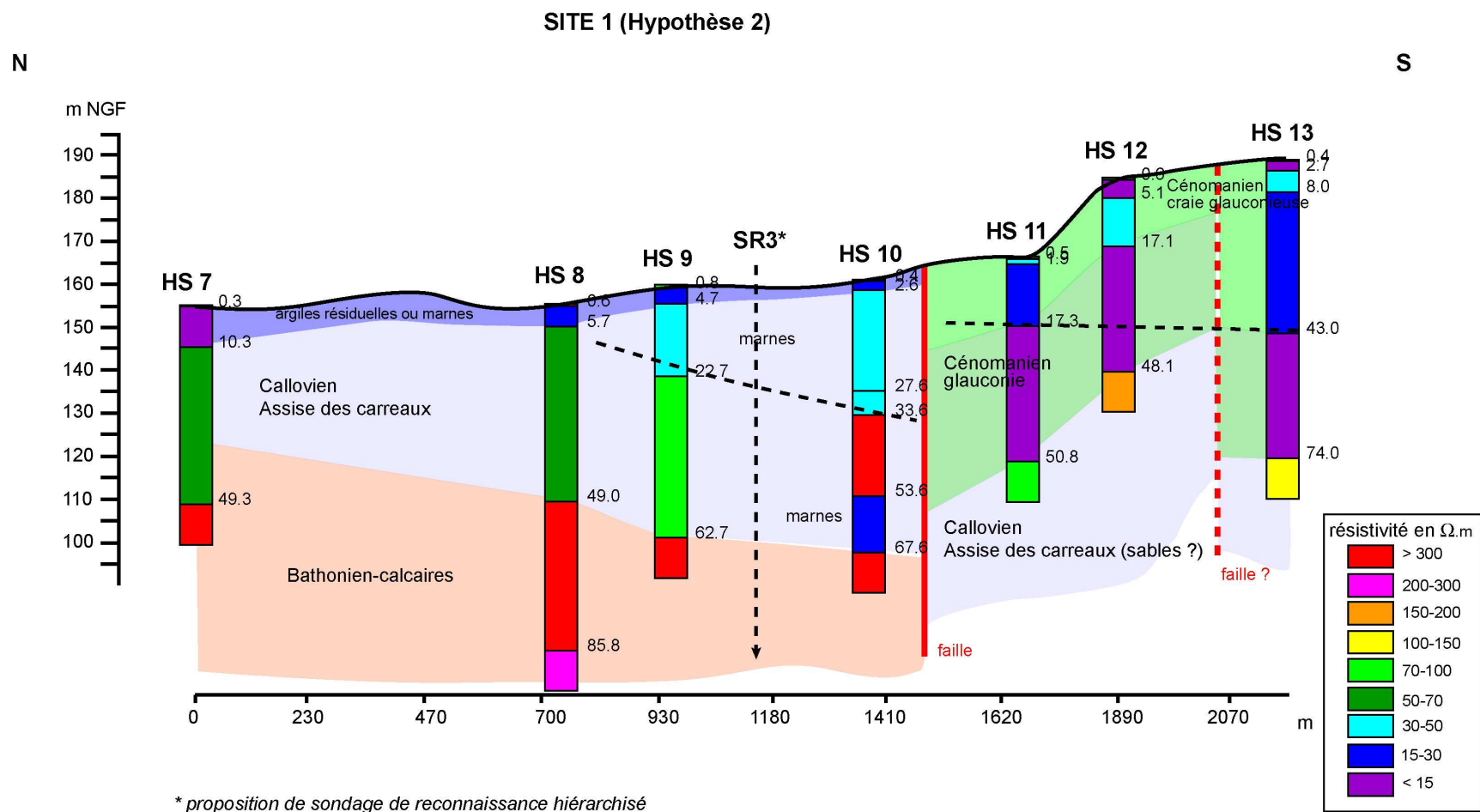
Fig. 16b : coupe interprétative du site 1 d'après les sondages électriques (hypothèse 2)
