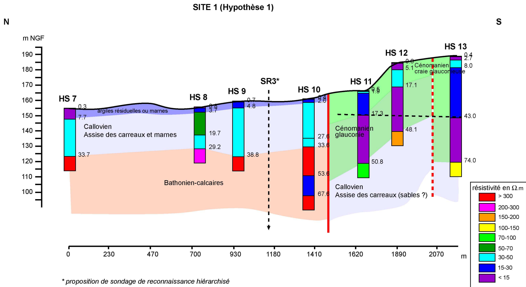
Fig. 16a : coupe interprétative du site 1 d'après les sondages électriques (hypothèse 1)
