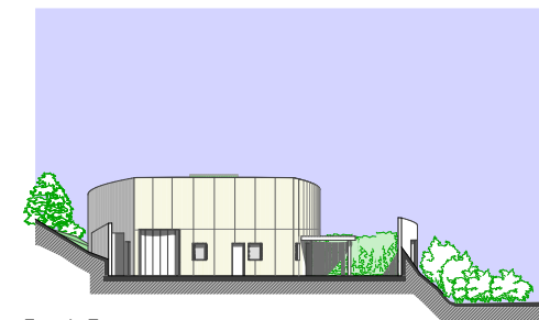
Façade Est 1/200
