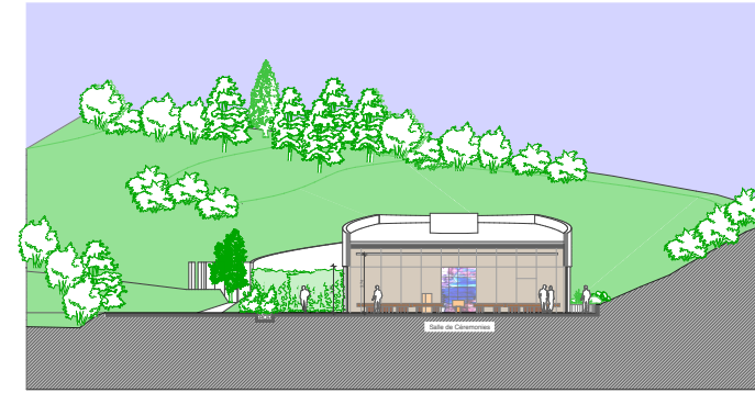
Coupe transversale 1/200
