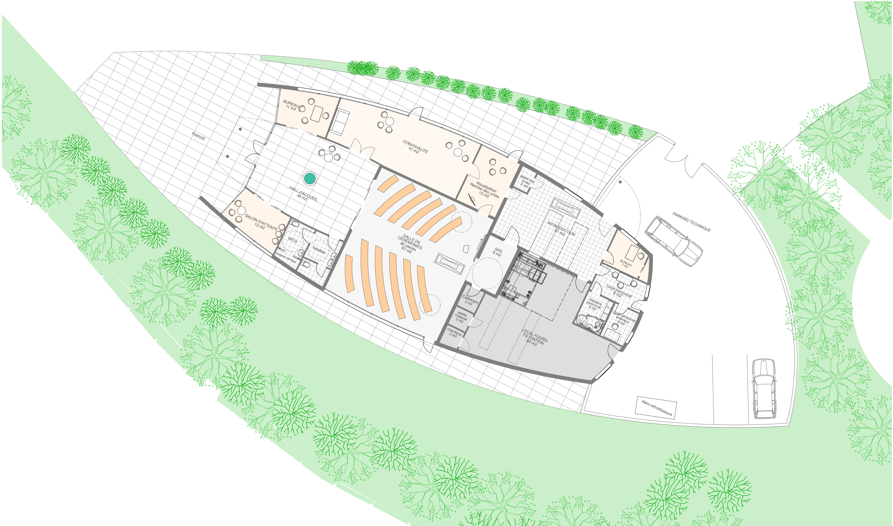
GRUPE BERTHELOT - CONSTRUCTION DU CREMATORIUM ET DU SITE CINERAIRE DES ANDELYS - PLAN DU BATIMENT
