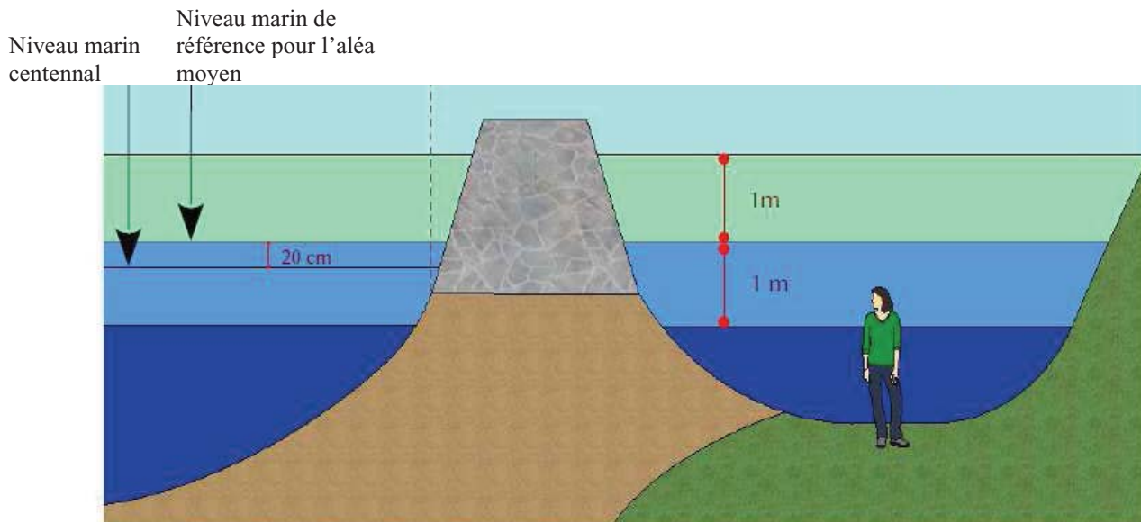
Illustration 7: Schéma de principe des zones sous le niveau marin (cas de la carte de l'événement moyen avec prise en compte de 20cm pour le changement climatique (identique au porter-à-connaissance (PAC) ZNM))
