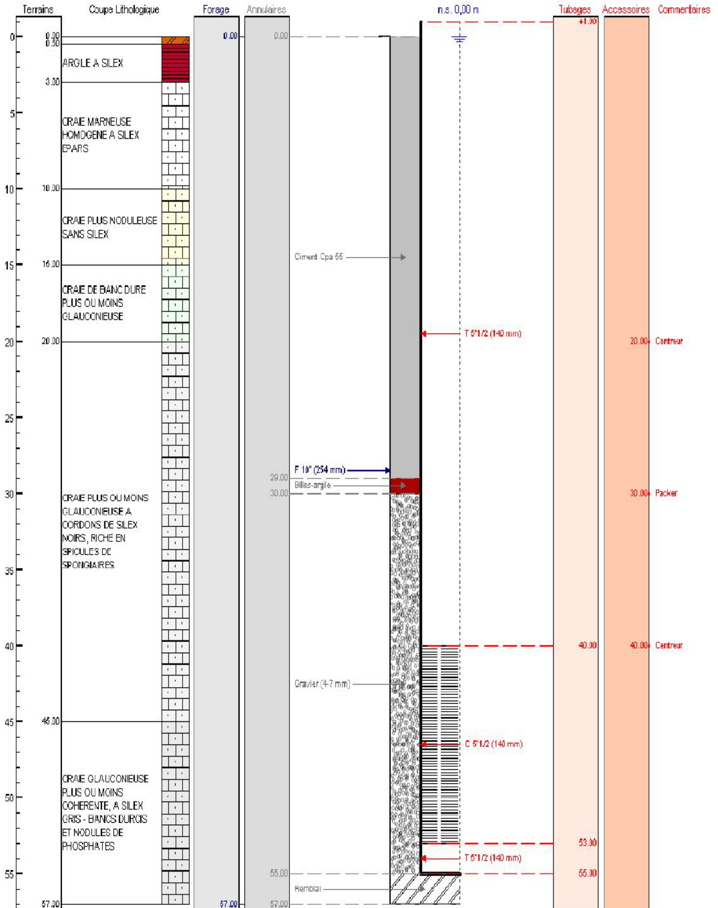
Coupe géologique & technique prévisionnelle du forage projeté par le G.A.E.C. LES JARDINS DU TORMELLIER au lieu-dit du TORMELLIER (SAINT-PIERRE-DE-CORMELLES - 27)
