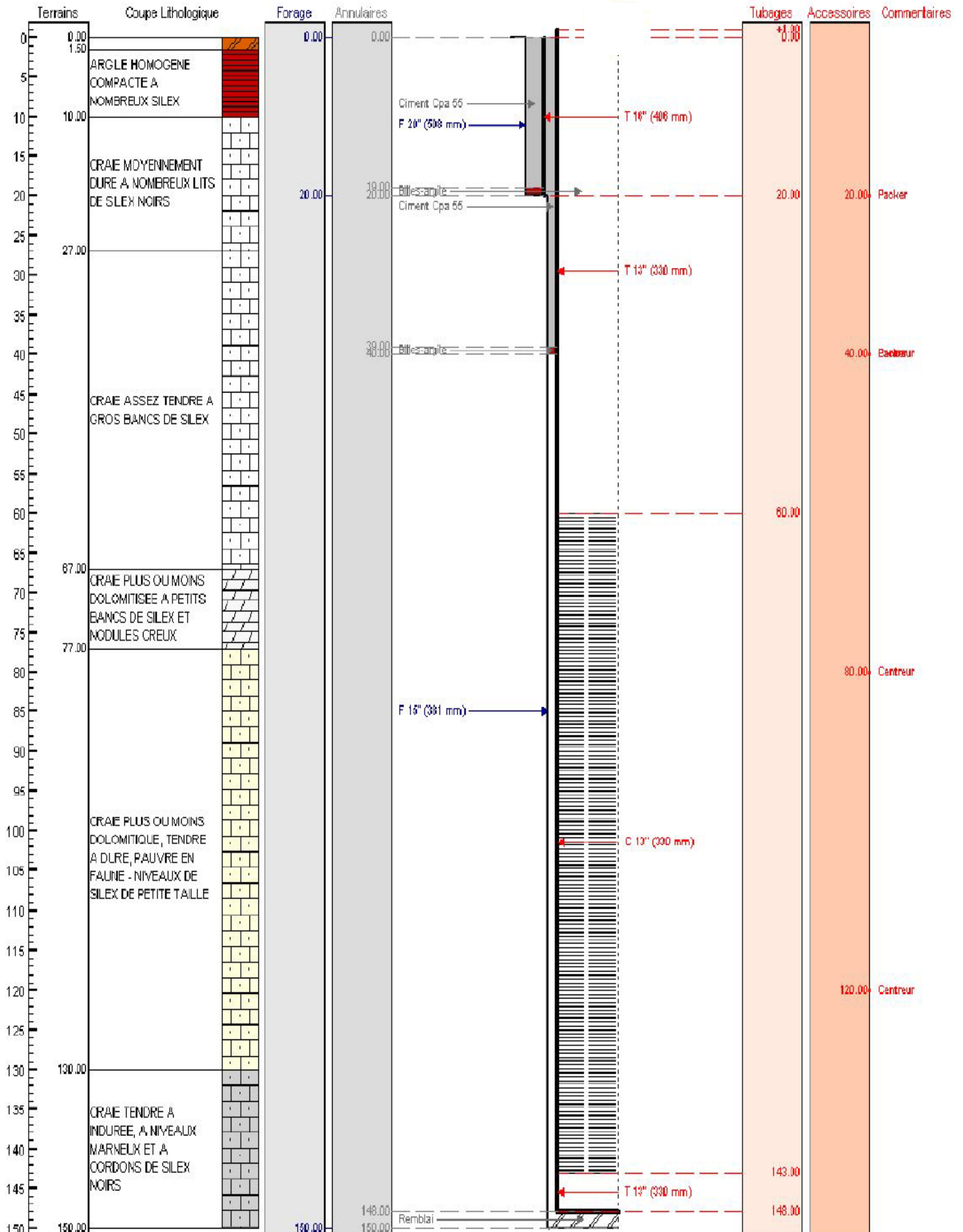
Coupe géologique & technique prévisionnelle du forage F1 projeté par la S.C.E.A. DU HAUT BECQUET au CLOS DE SAINT-PIERRE BOUVRY (FARCEAUX - 27)
