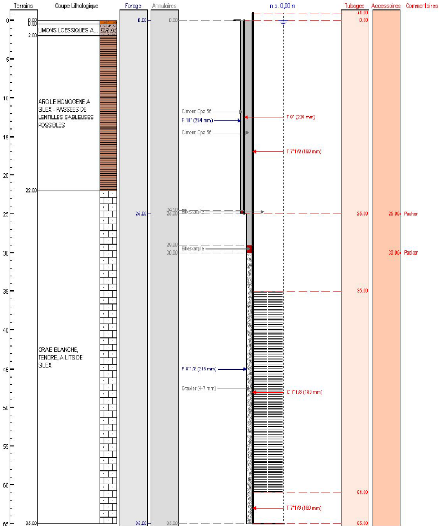
Coupe géologique & technique prévisionnelle des sondages projetés à INGOUVILLE (76)
