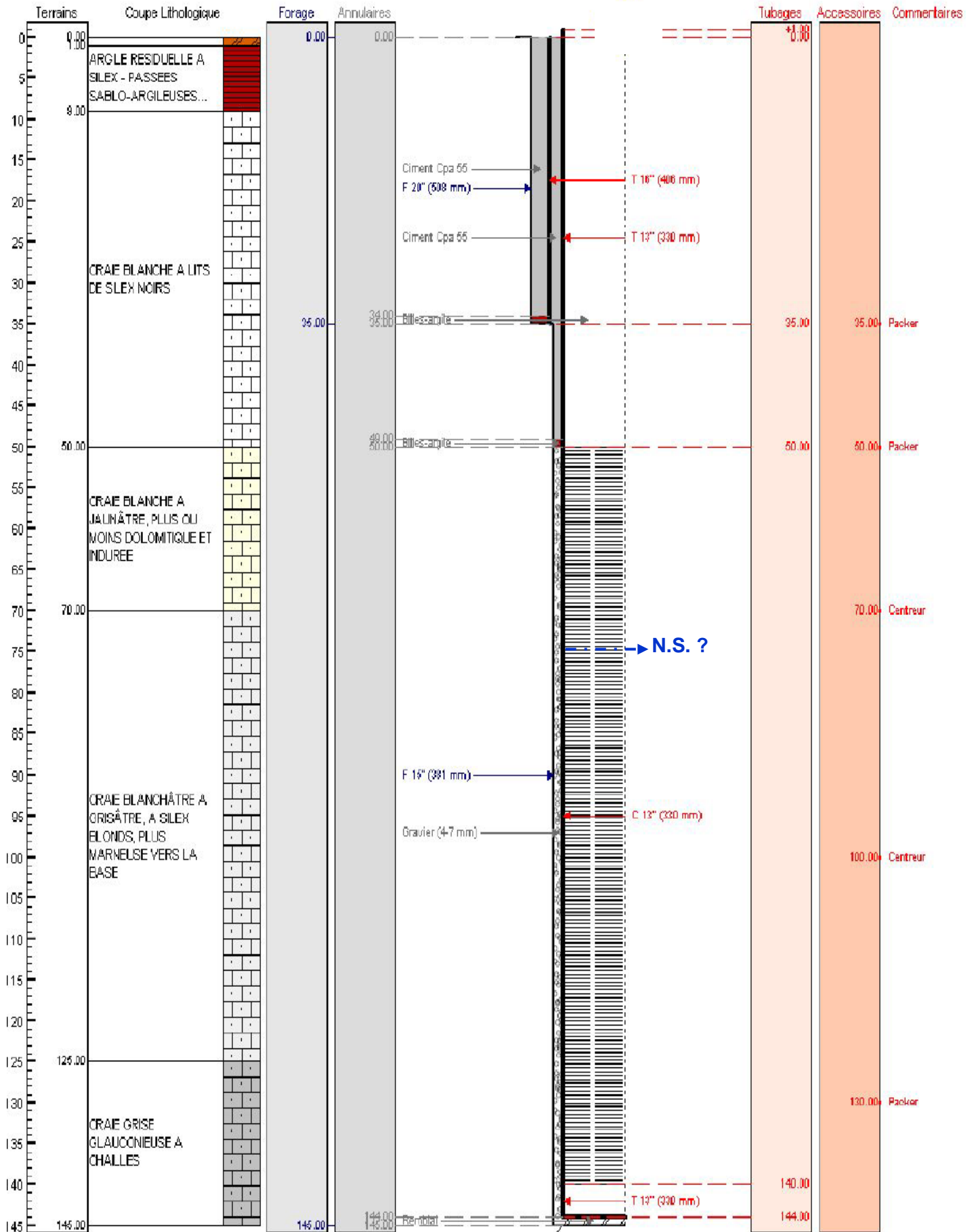
Coupe Géologique et Technique prévisionnelle du forage projeté à LA FOSSE AU GROS sur le territoire de la commune de VENON (27)
