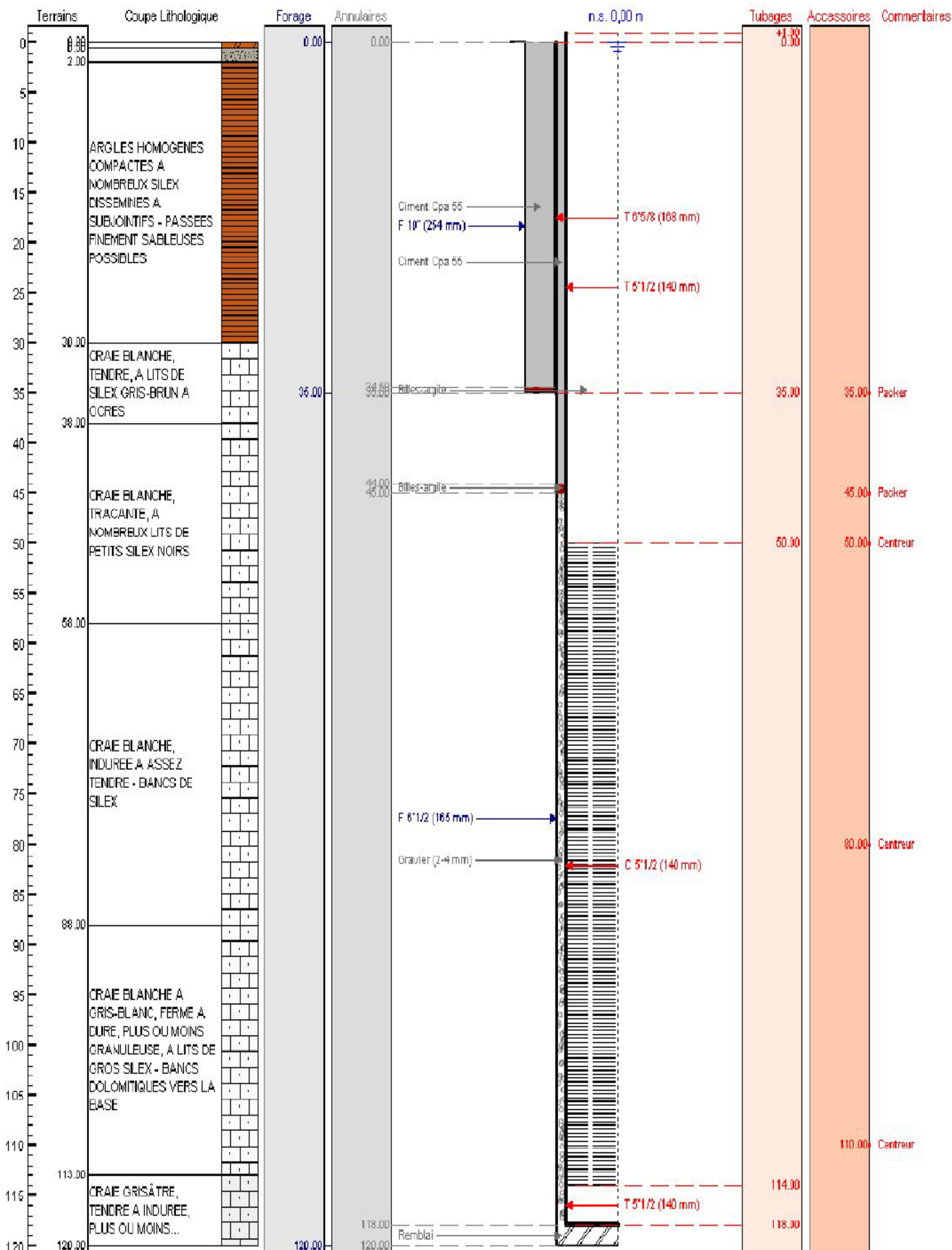
Coupe Géologique et Technique prévisionnelle du forage projeté à BACQUEPUIS (27)
