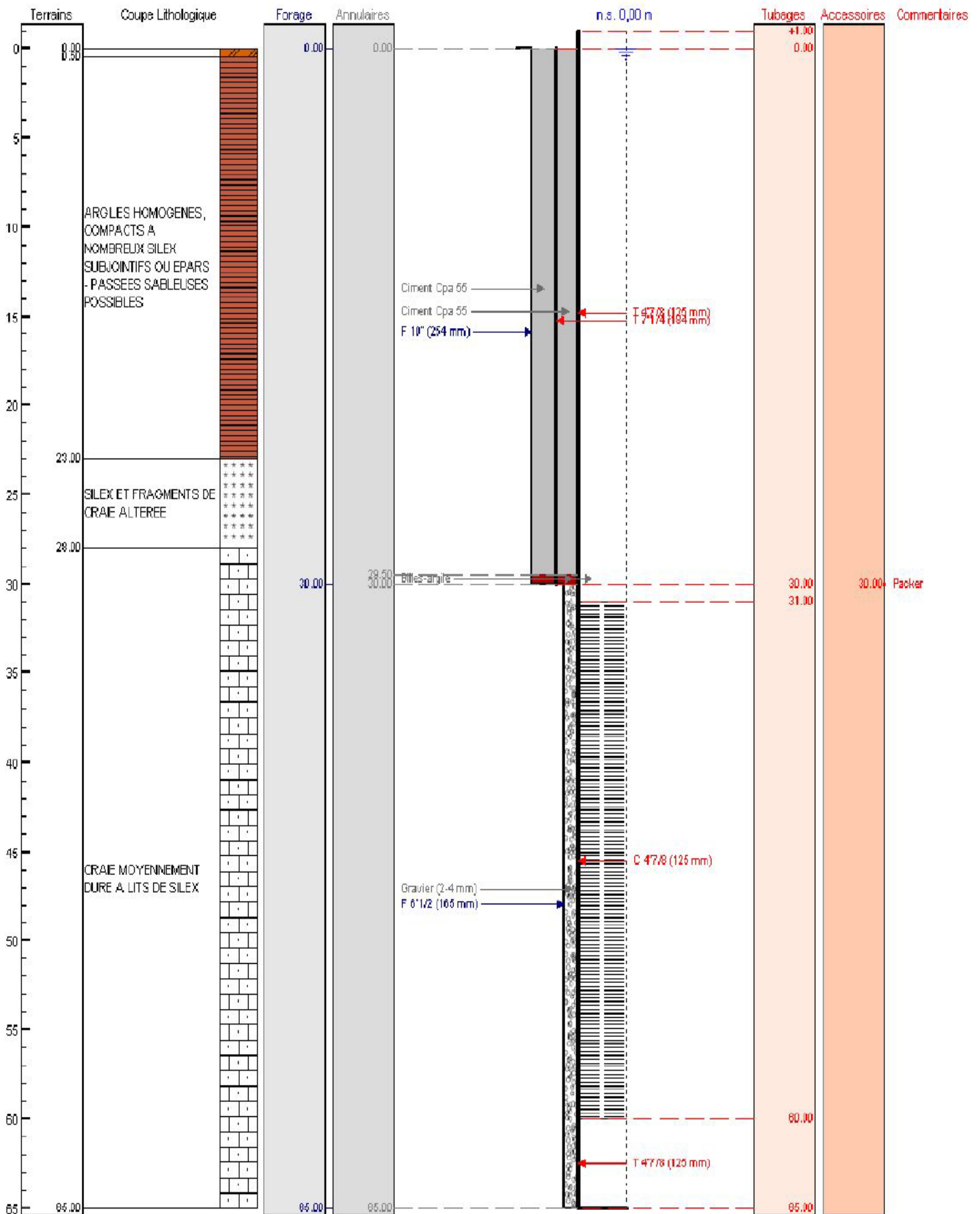
Coupe Géologique et Technique prévisionnelle du forage projeté à PISEUX (27)
