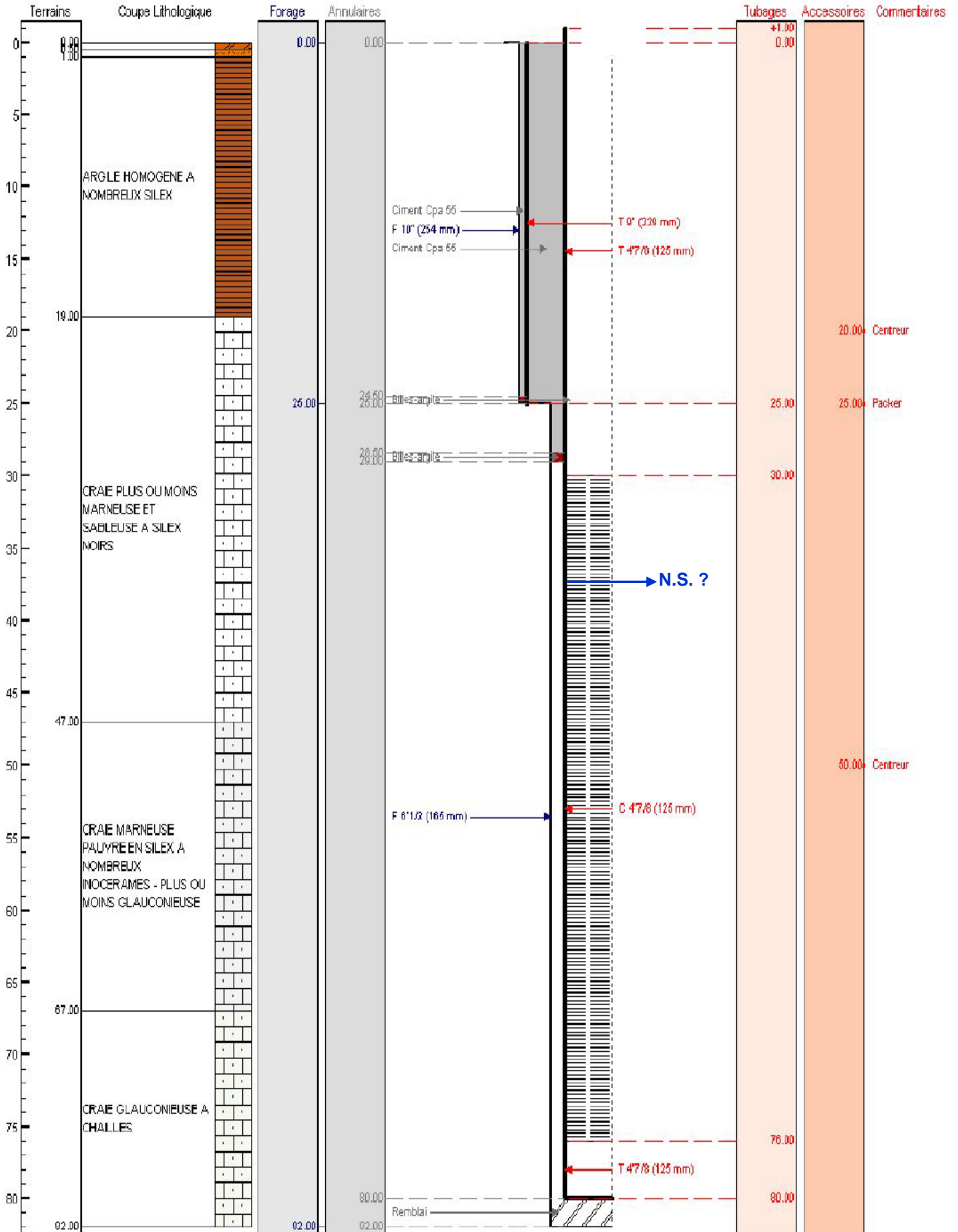
Coupe géologique & technique prévisionnelle du forage projeté par le G.A.E.C. VANDERMEERSCH à LA SOIZIERE (GRAND-CAMP - 27)
