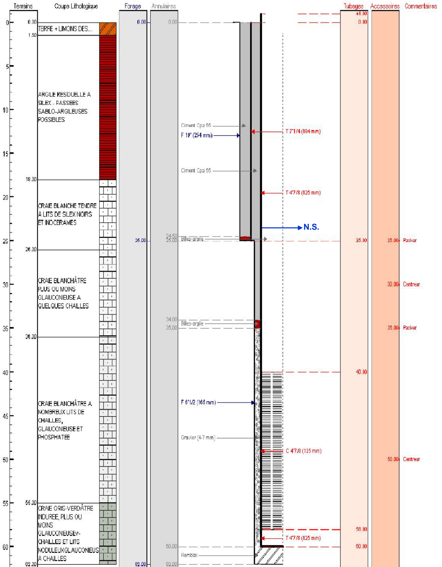
Coupe géologique & technique prévisionnelle du forage projeté à LA CONARDIERE (SAINT-AUBIN-DU-THENNEY - 27)
