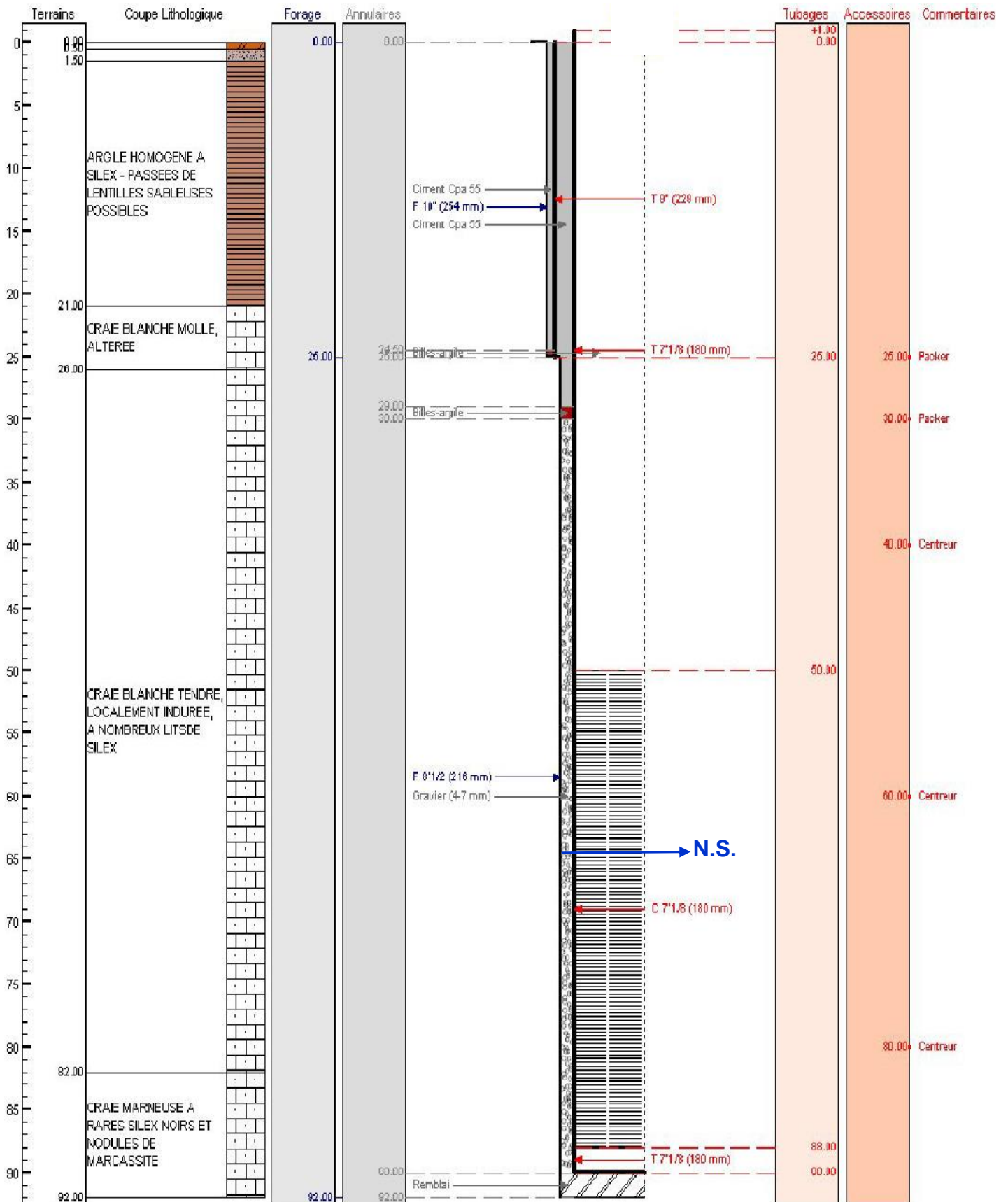
Coupe géologique & technique prévisionnelle du forage F1 projeté par l'E.A.R.L. DE LA CROIX MAHIEU près du « CHÂTEAU » à INGOUVILLE (76)
