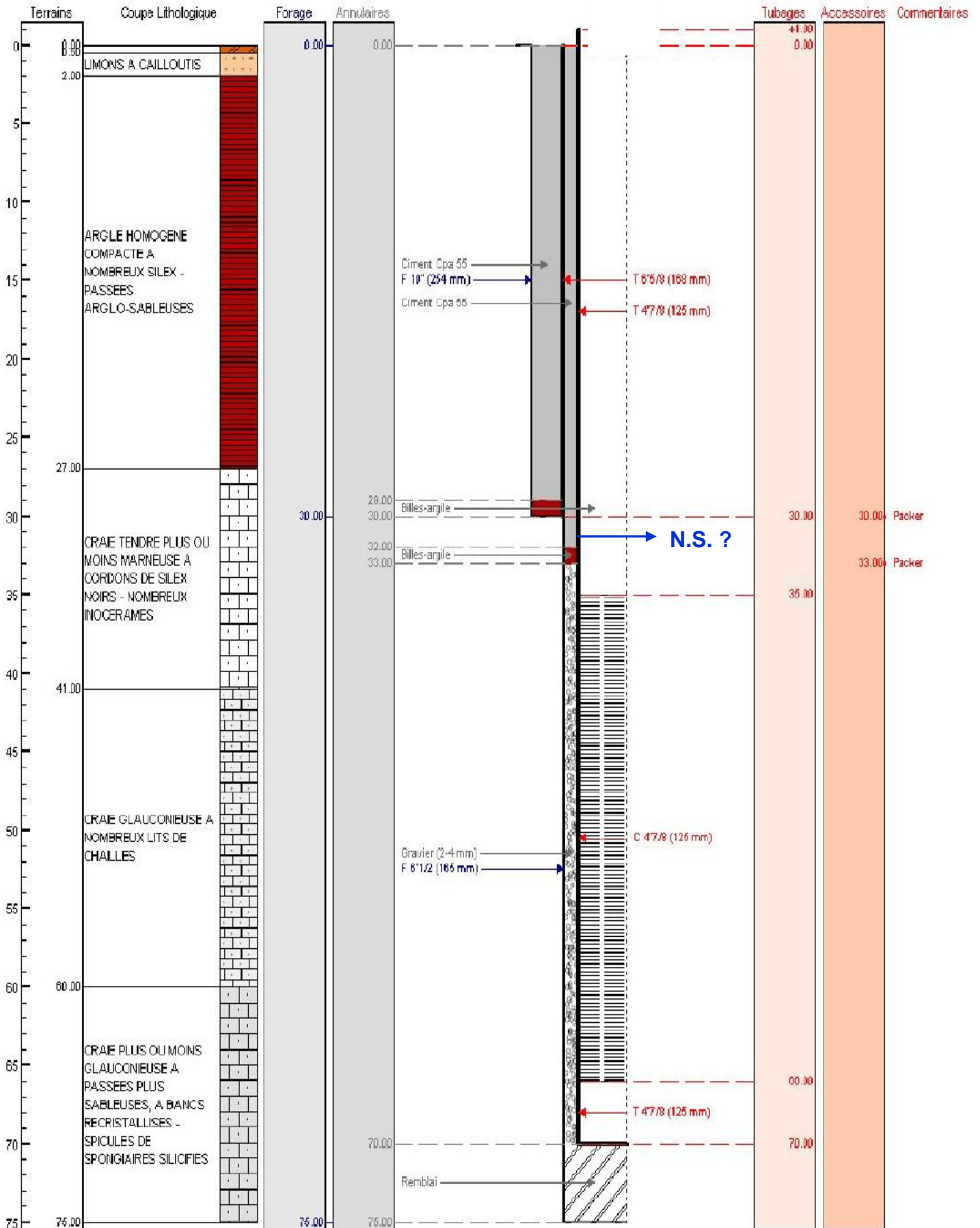
Coupe Géologique et Technique prévisionnelle du forage projeté aux NOES (SAINT-AGNAN-DE-CERNIERES - 27)
