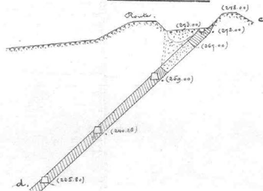
Figure 21 : Effondrements localisés de type fontis par rupture du toit (La Ferrière-aux-Etangs, effondrement de 1906, document d'archives, 1906)
