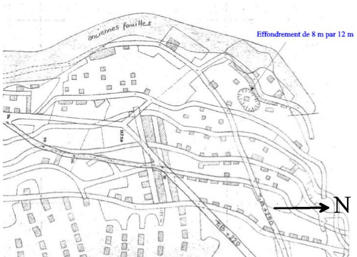
Figure 22 : Effondrement de La Fieffe du 8 mai 1974. Position de l'effondrement par rapport aux travaux du fond (plan au 1/1000 ème )
