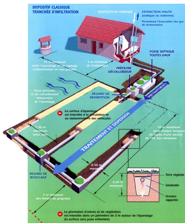
Figure 1 : principes des systèmes d'assainissement non collectif
