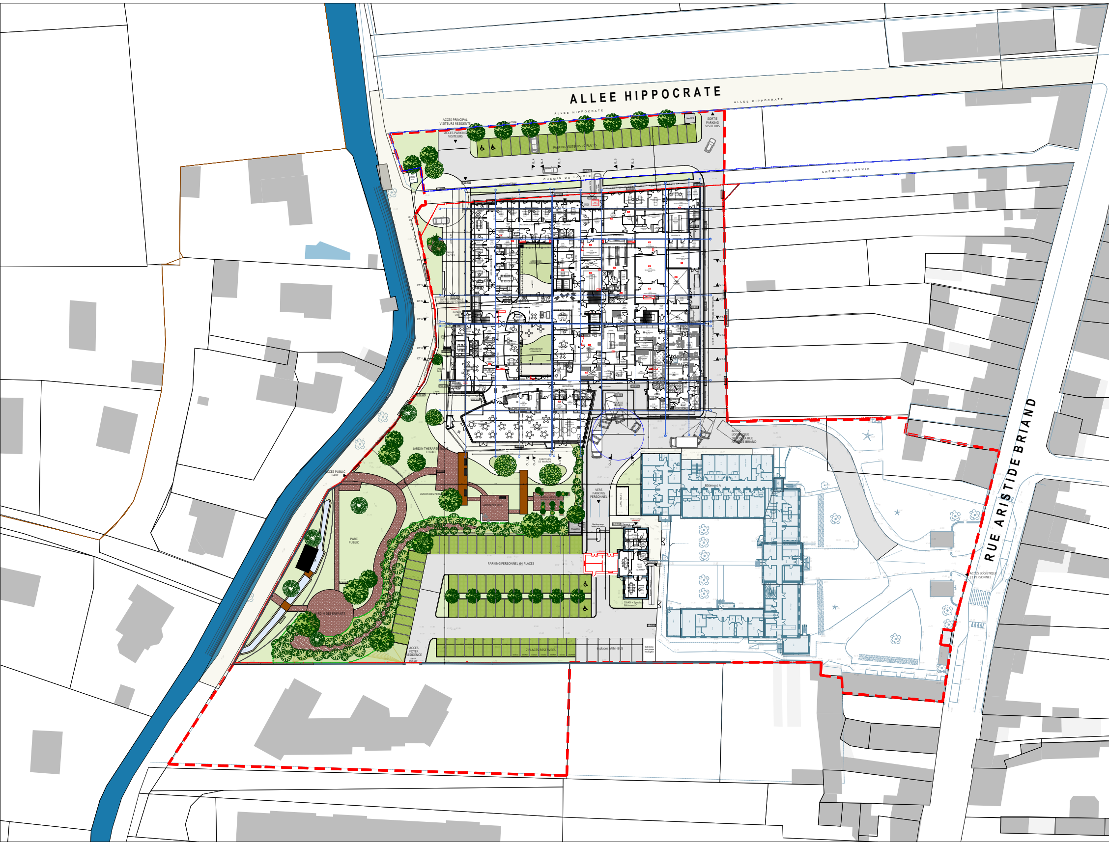
EXTRAIT DE PLAN PROJET - NIVEAU RDC
